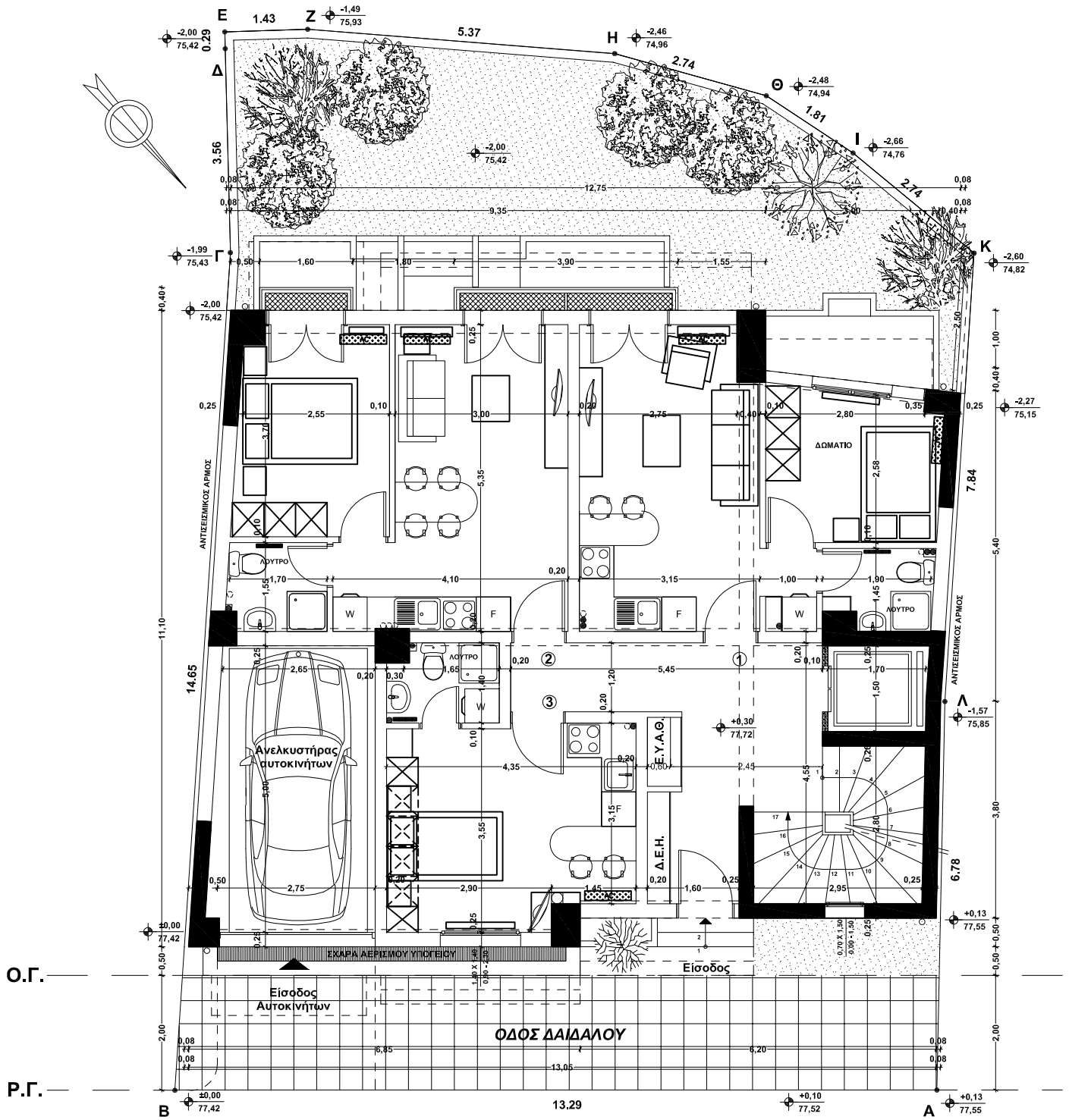
ΚΑΤΟΨΗ ΙΣΟΓΕΙΟΥ ΔΙΑΜΟΡΦΩΣΗ ΑΚΑΛΥΠΤΟΥ ΚΛ. 1:100
